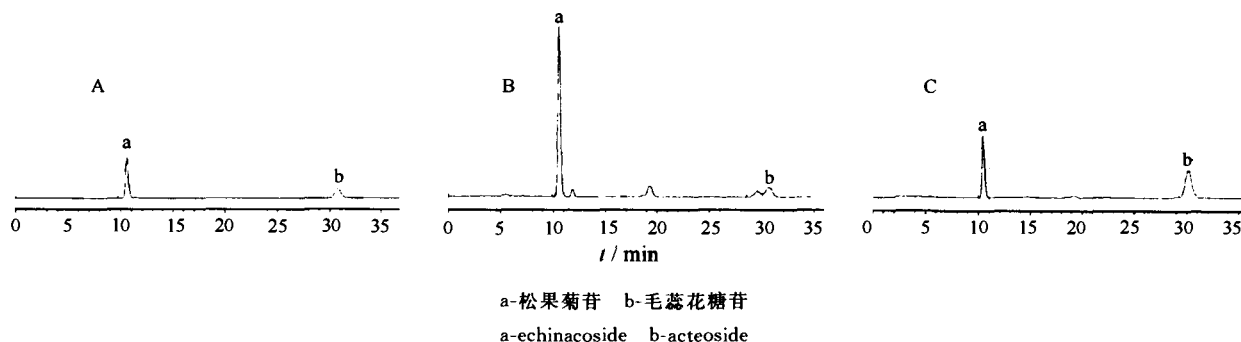
图 2 松果菊苷和洋丁香苷(毛蕊花糖苷)对照品(A)、肉苁蓉愈伤组织(B)、野生肉苁蓉(C)的 HPLC 图谱
