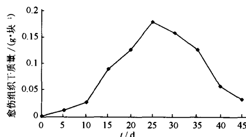
图 1 肉苁蓉愈伤组织生长曲线
